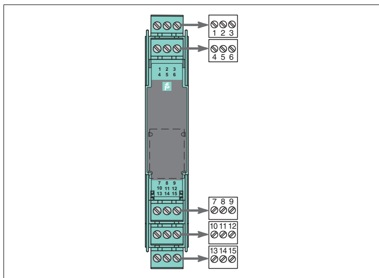
Рис. 2.9 Корпус устройства КФ (корпус 20 мм)
