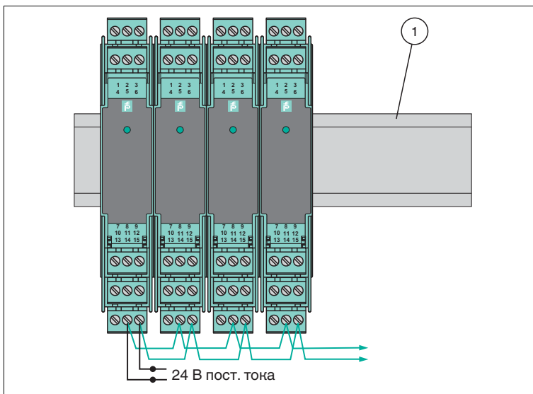
Рис. 3.5 Стандартная установка
