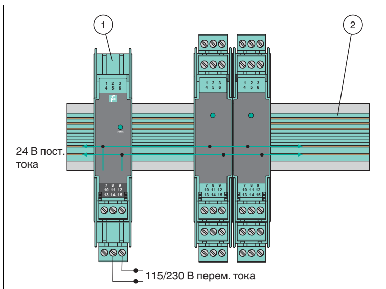
Рис. 3.9 Встроенный источник питания (500 мА)
