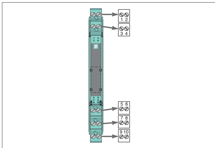
Рис. 2.8 Корпус устройства КС (корпус 12,5 мм)
