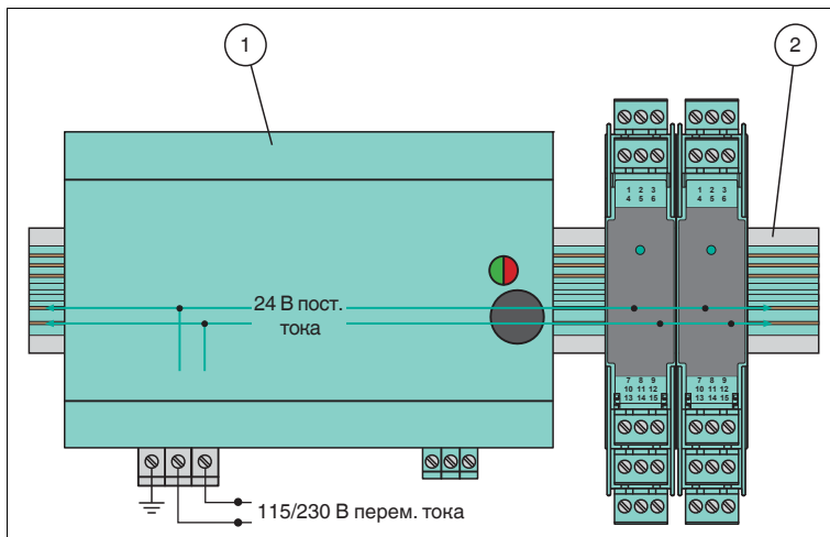
Рис. 3.8 Встроенный источник питания (4 А)
